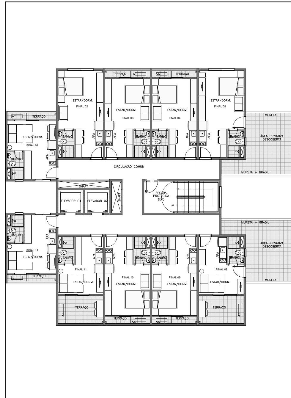
4º PAVIMENTO
