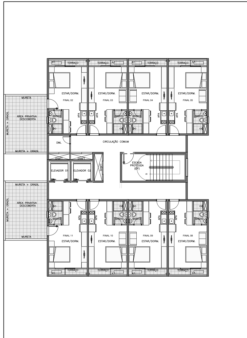
9º PAVIMENTO
