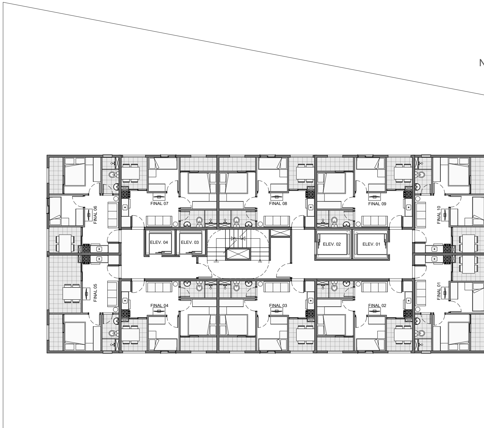
5° AO 12° PAVIMENTO sem escala
