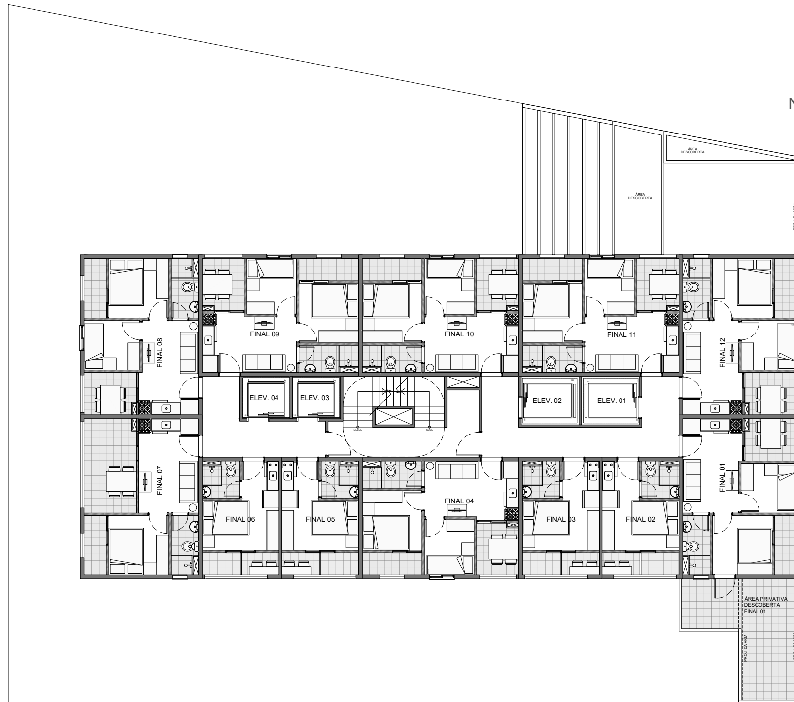
1º PAVIMENTO sem escala
